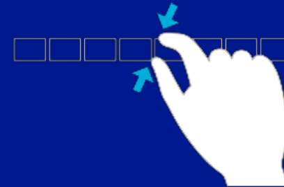
Zoom sémantique
