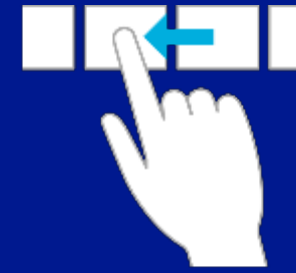
Défilement
